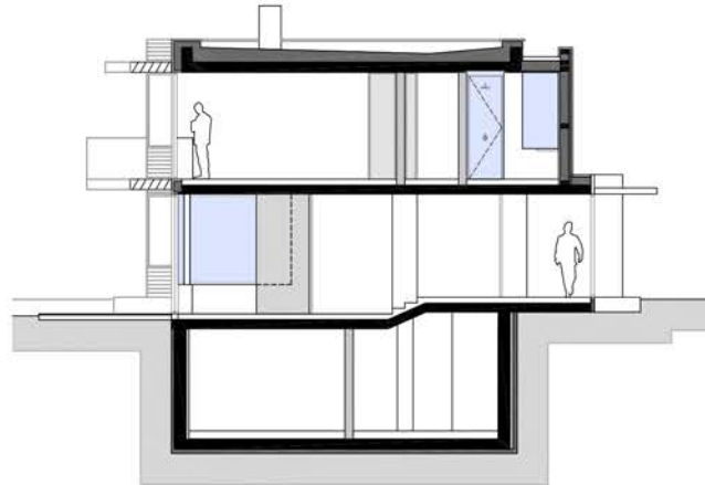
Schnit II 1:200
