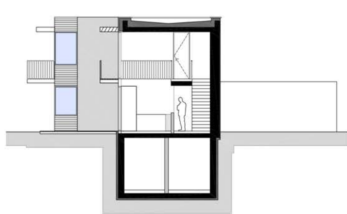
Schnit I 1:200
